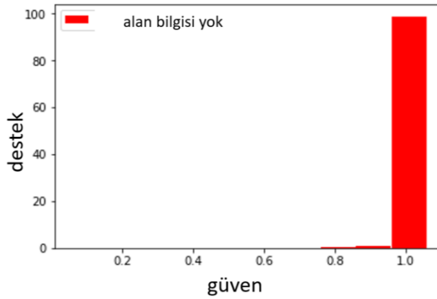
Şekil 5. Deney A kurallar yüzdesi – güven.
